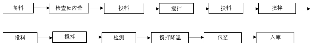
图 3 厌氧胶生产工艺流程图
