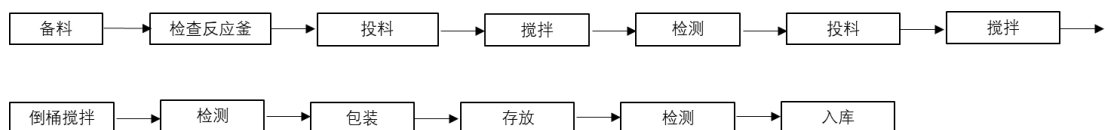
图 5 三防漆生产工艺流程图
